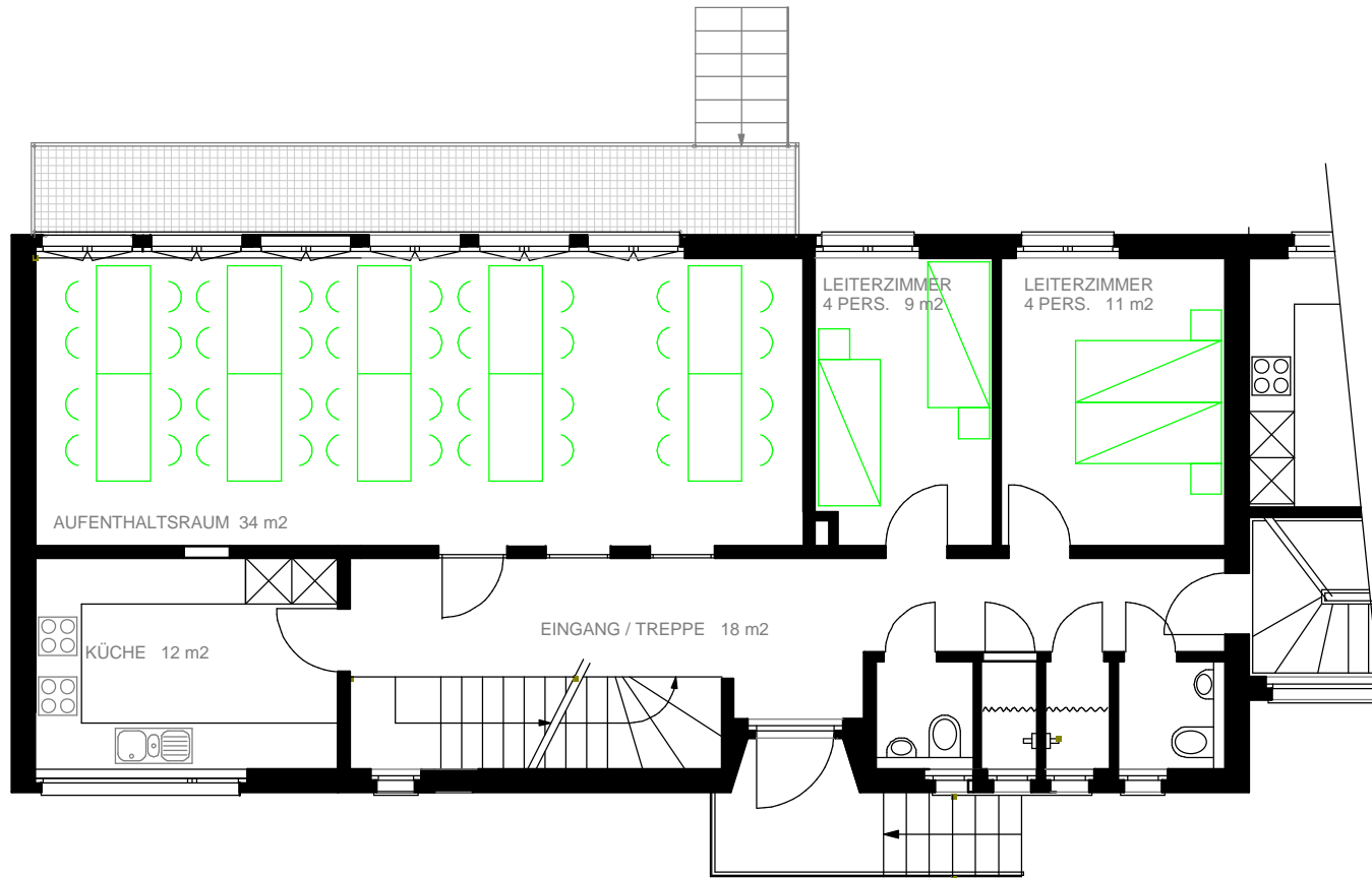
GRUNDRISS ERDGESCHOSS
